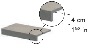
16,5x30 . 6 1/2 "x12" ELEMENTO A L MONOLITICO G3SO05ELM HSO 5
